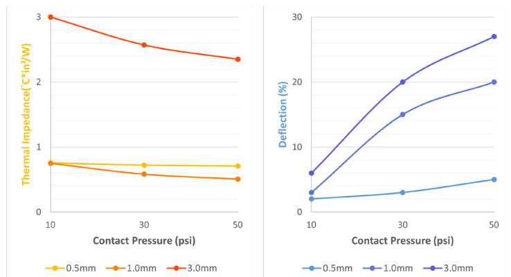
壓力, 熱阻抗, 變形量示意圖
