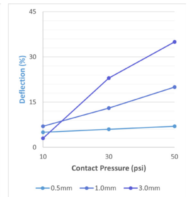
壓力，熱阻抗，變形量示意圖
