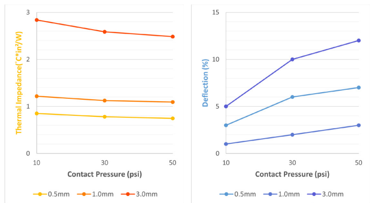
压力, 热阻抗, 变形量示意图
